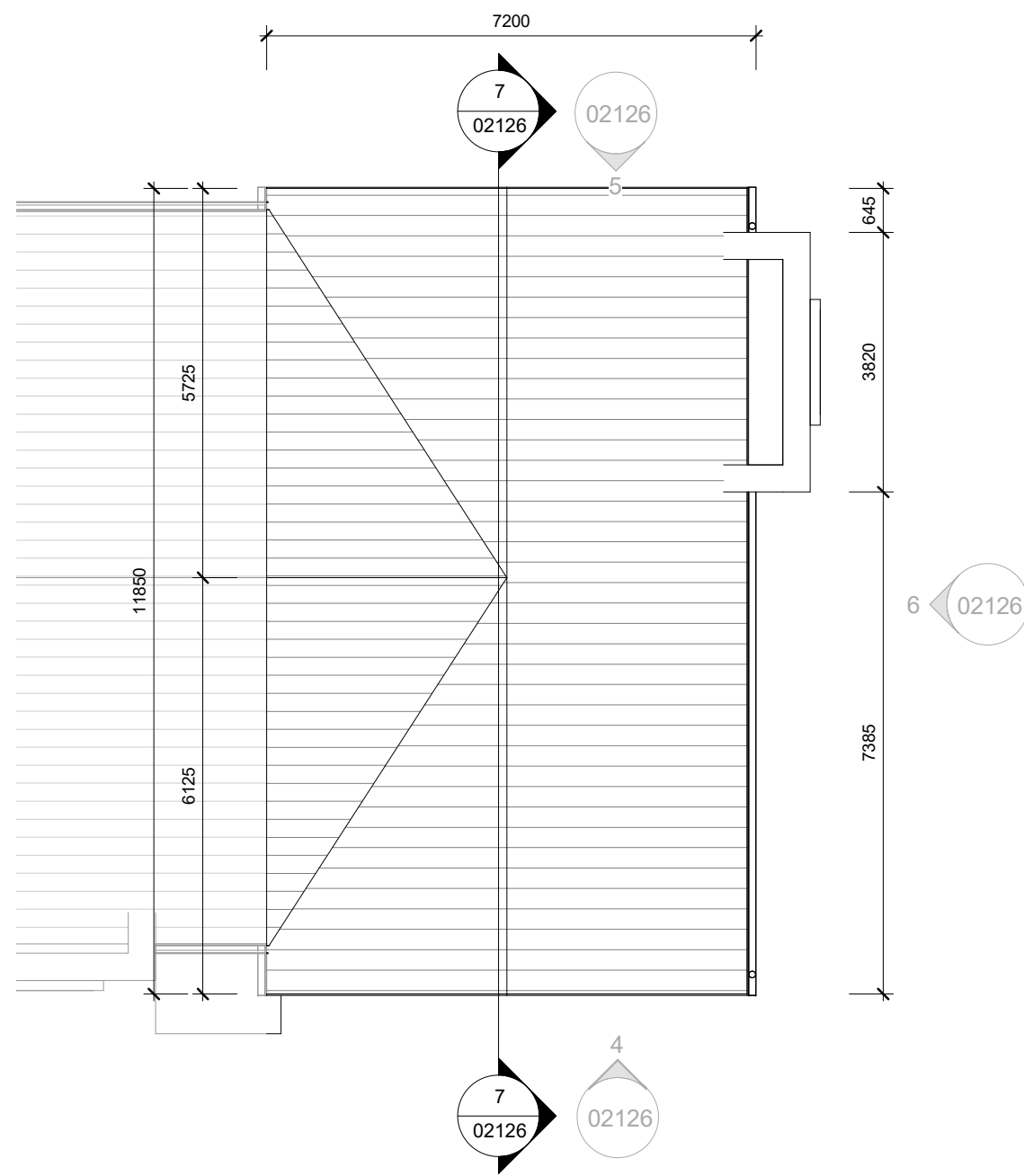
3 ROOF PLAN 1 : 100
